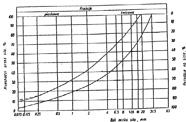
Rys. 1. Pole dobrego uziarnienia kruszywa dla podbudowy
